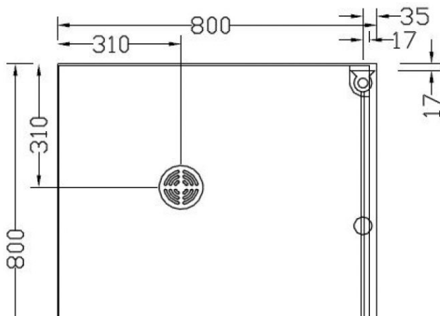
Eckduschwanne 1010
