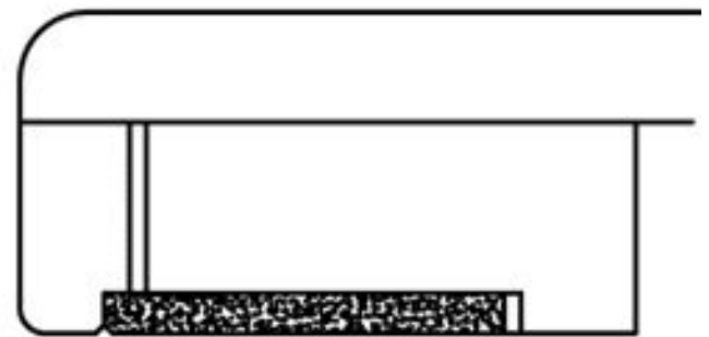
mit Creanit geschlossene Unterseite und Tropfnase
