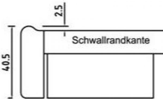
Kante mit Schwallrand
