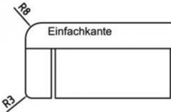
Kante Standard
