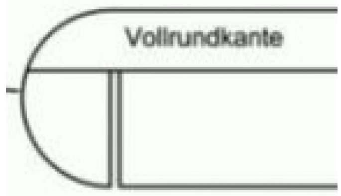
Kante vollrund
