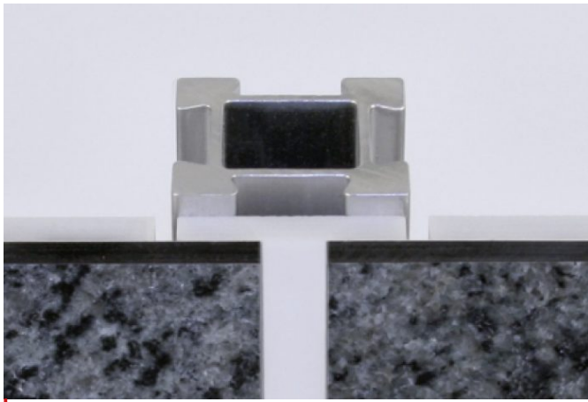
Naturstein-Front (Horizontalschnitt)
