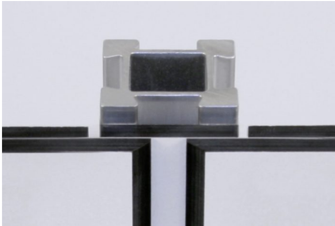
HPL-Front Schwarzkante gefräst (Horizontalschnitt)
