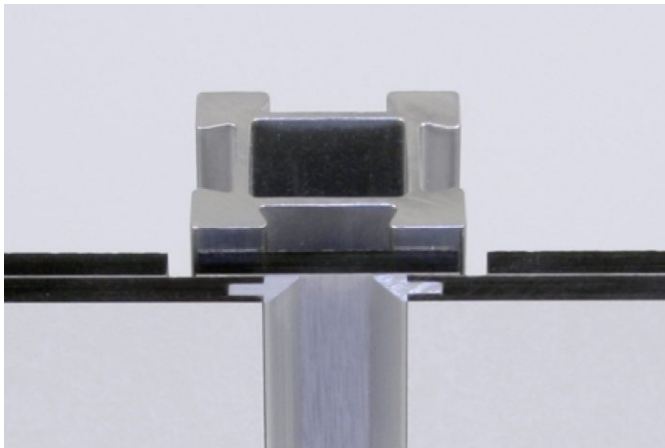
HPL-Front Alukante (Horizontalschnitt)
